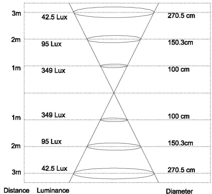
WL55-16-12 double face 2 fois 3LED 1W (I= 0,5A) Idéal pour éclairage de couloir, entrée, escalier. Diam 50 x L 116mm
